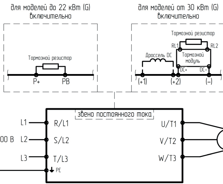
Рисунок 3. Подключение силовых клемм
